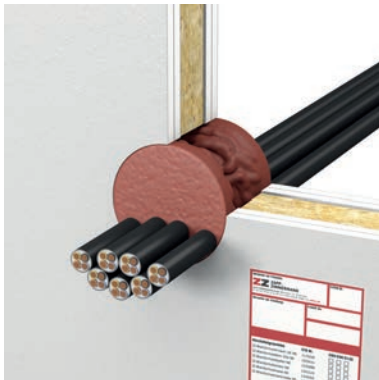
ZZ Brandschutzmasse NE LTW
