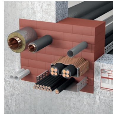
ZZ 230 Brandschutzstein MW
