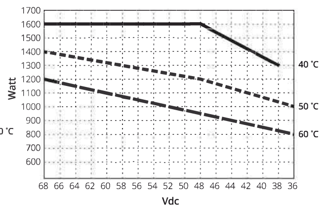
SR-1600 PLUS - 148 / 248:
