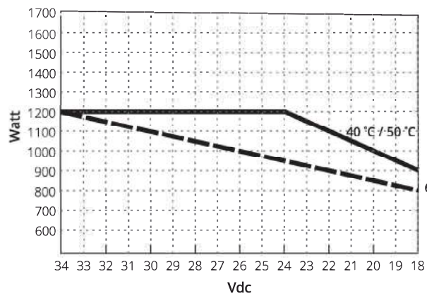
SR-1600 PLUS - 124 / 224:
